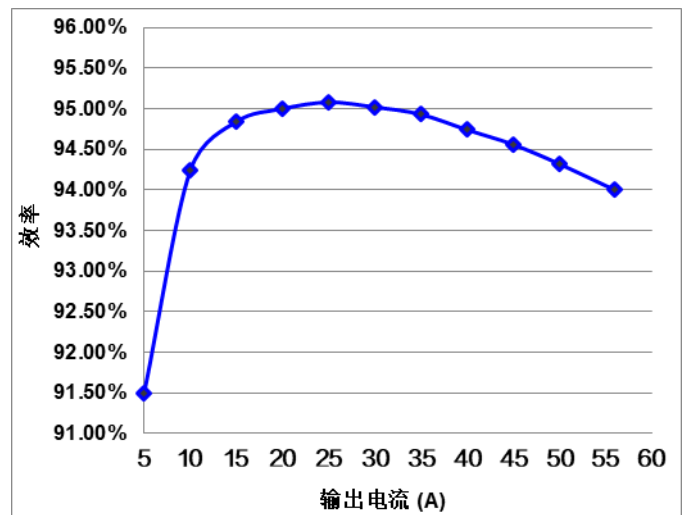
图2 输出效率曲线图 (Vout = 53.5V DC, Ta = 25℃)
