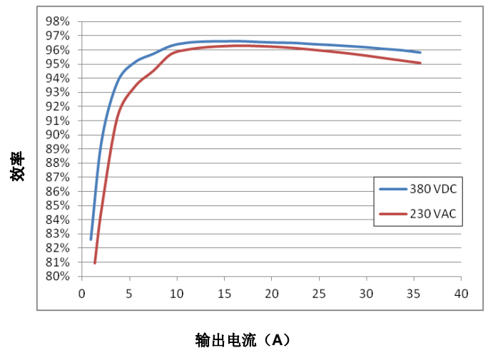
图2 输出效率曲线图 ( V_{out}=53.5V , T_a: 25^\circ C )
