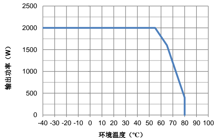
图3 功率降额曲线
