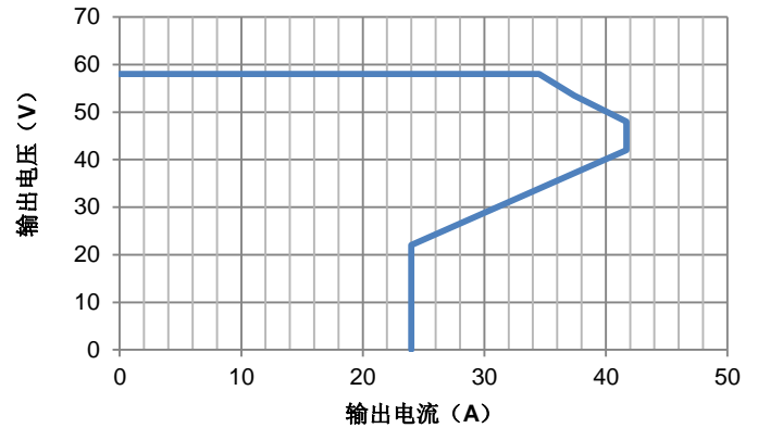
图1 输出外特性曲线图
