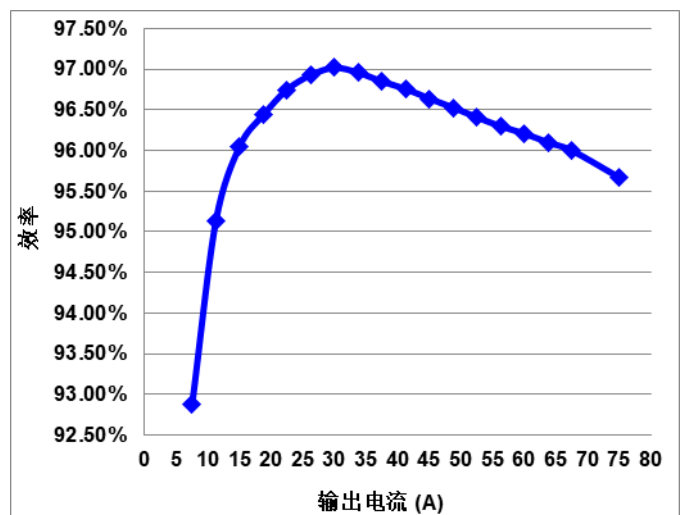
图2 输出效率曲线 (230V AC, 25°C)
