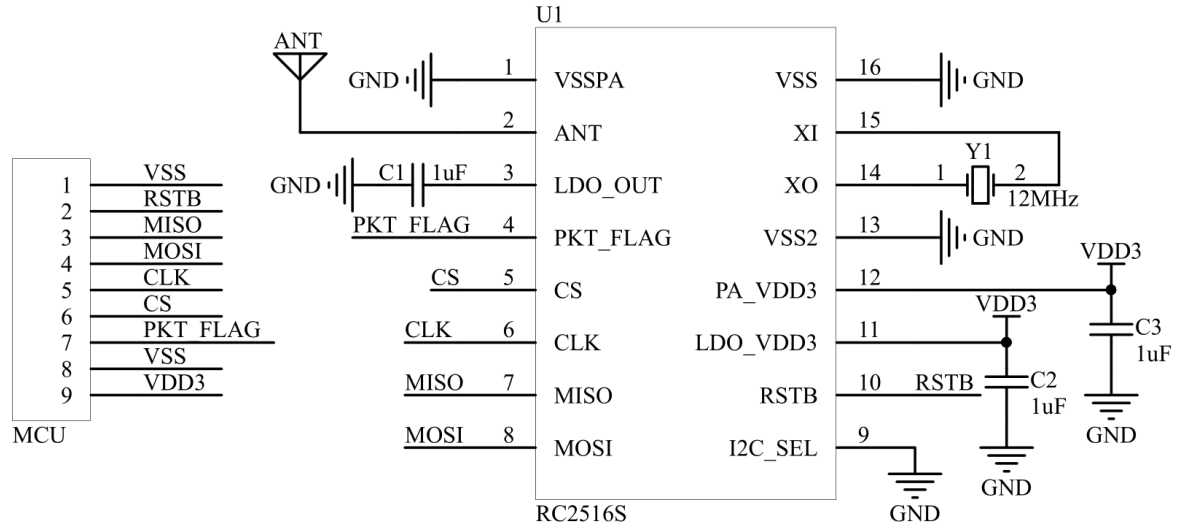
图 11.2 RC2516S（SPI）典型应用电路
