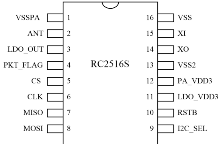
图5.1 RC2516S-SOP16 引脚定义图
