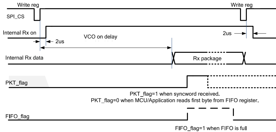
当 Reg0x01[2:1]='b00 or 'b01 时，RX 时序图
