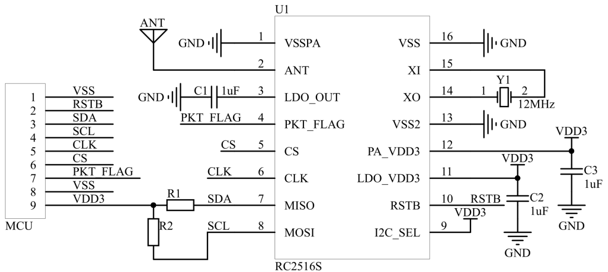
图 11.3 RC2516S（I2C 地址 A4=1）典型应用电路
