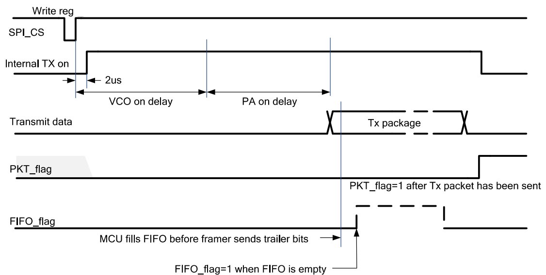
TX 时序图
