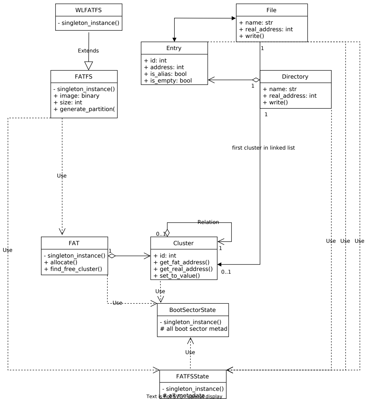
图 40: FAT 文件系统生成器及解析器设计架构
