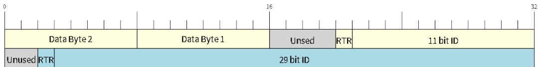
图 29: 单过滤器模式的位布局（右侧为最高有效位）
