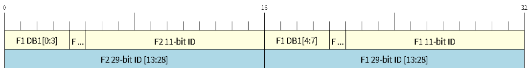
图 30: 双过滤器模式的位布局（右侧为最高有效位）
