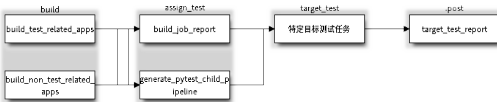
图 4: 目标测试子流水线工作流程
