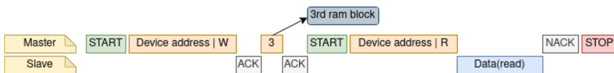
图 12: 从 I2C 从机 RAM 中获取数据
