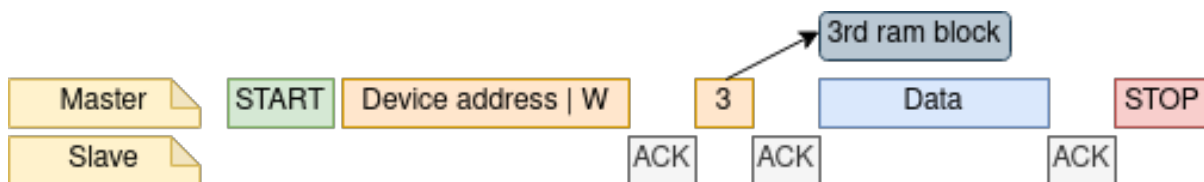
图 11: 将数据放入 I2C 从机 RAM 中
