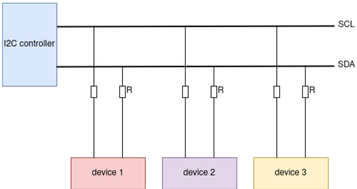
图 6: I2C 主机总线-设备模块
