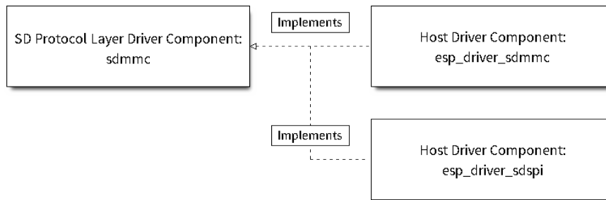
图 41: SD 主机端组件架构
