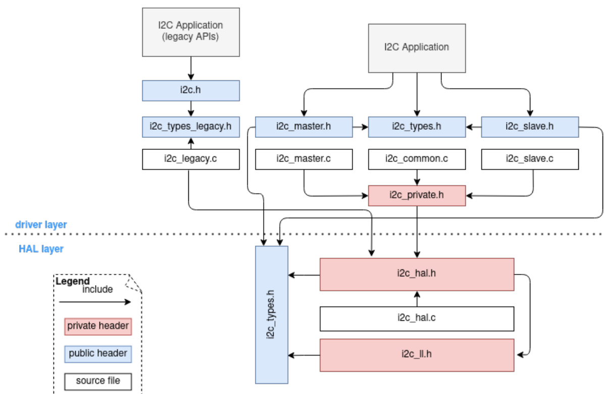
图 5: I2C 文件结构
