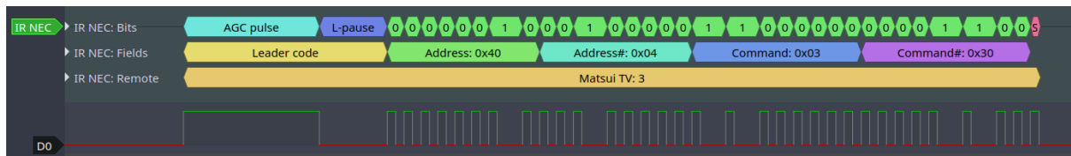
图 24: 红外 NEC 帧
