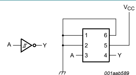
Fig. 10. Inverter
