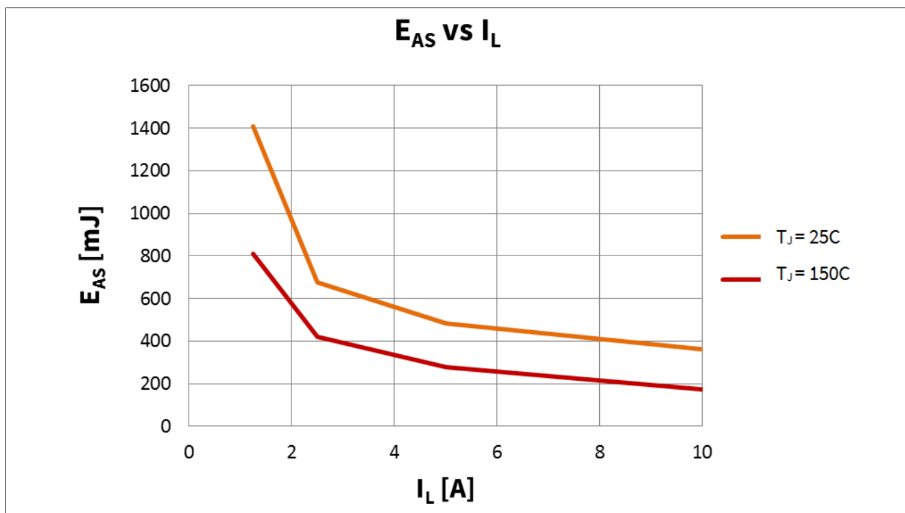
Figure 29 E_{AS} vs. I_L @ T_{J(0)}=25^\circ\text{C} , 150^\circ\text{C} , V_{BAT}=13.5\text{V} ; V_{IN} = V_{ENABLE} = V_{DD} = \text{open} ; I_L = I_{L(NOM)}/4 , I_{L(NOM)}/2 , I_{L(NOM)} , 2 \cdot I_{L(NOM)}
