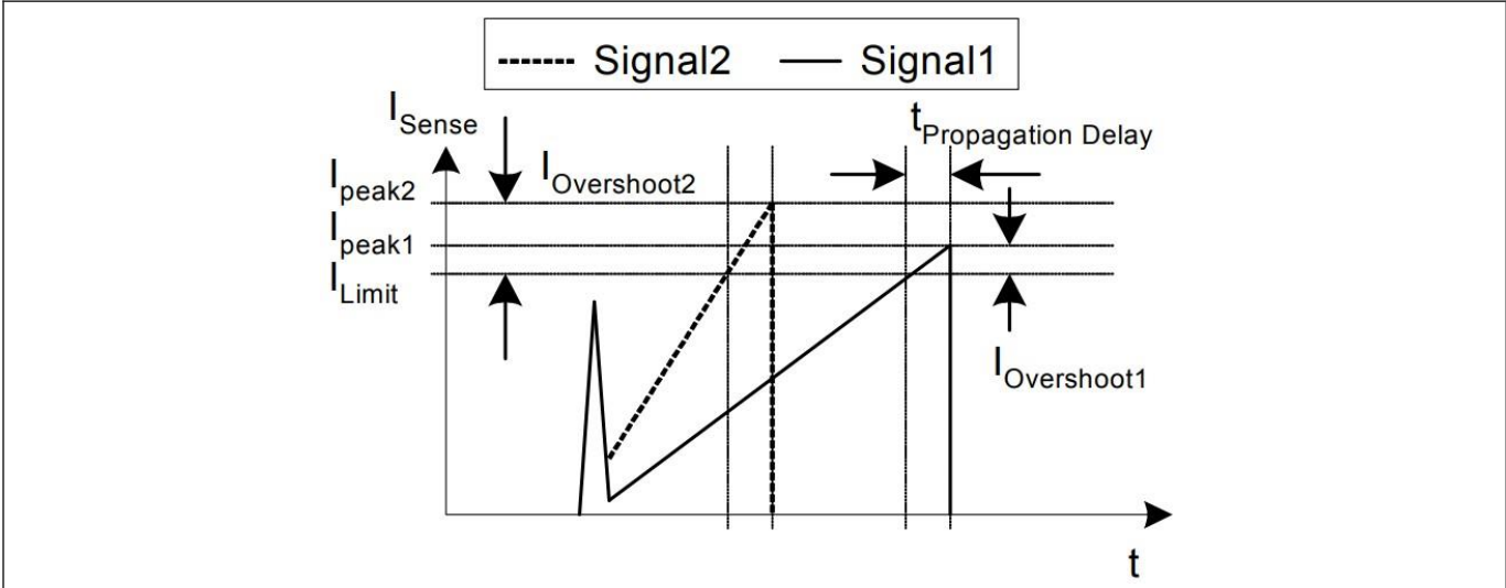
图 10 限流
