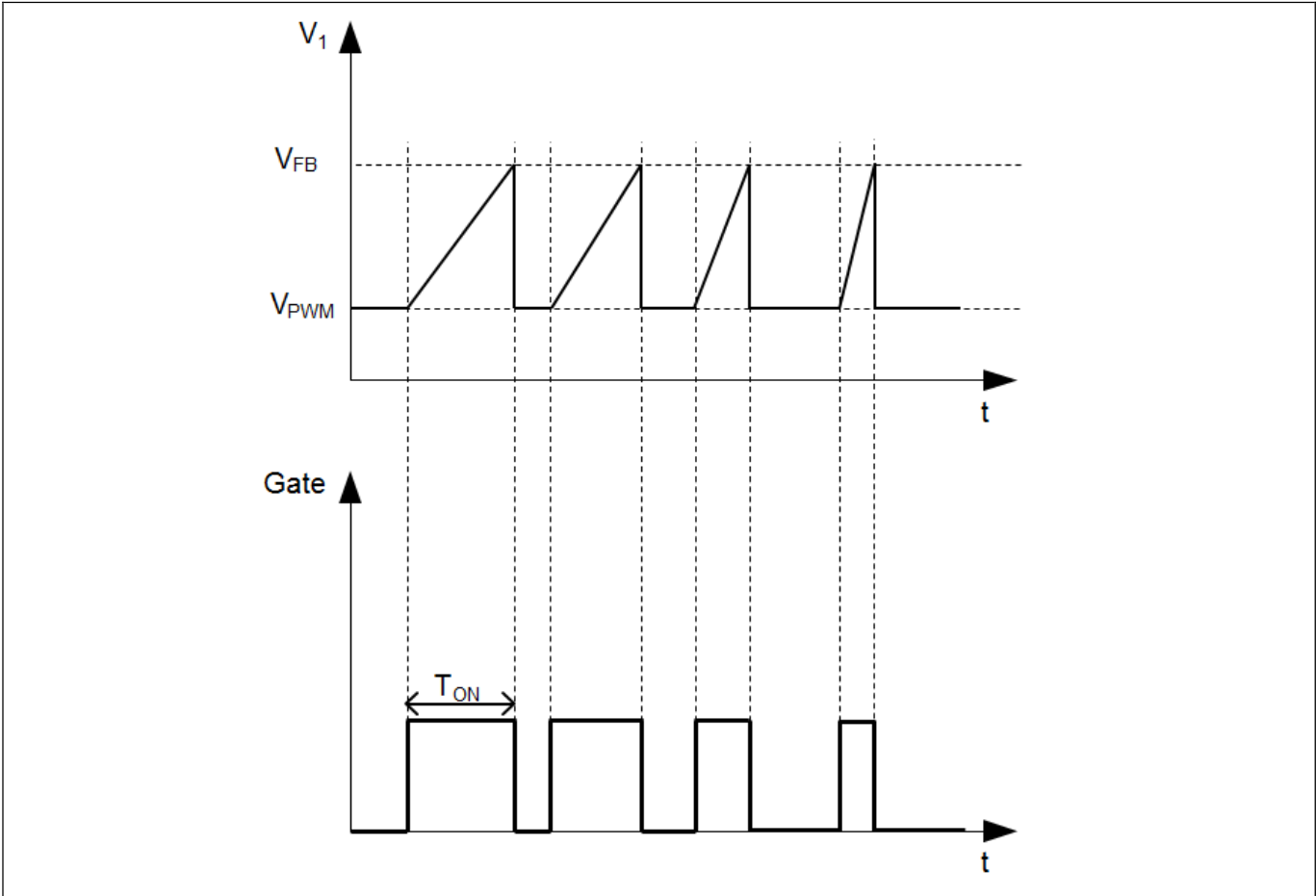
图 7 脉宽调制
