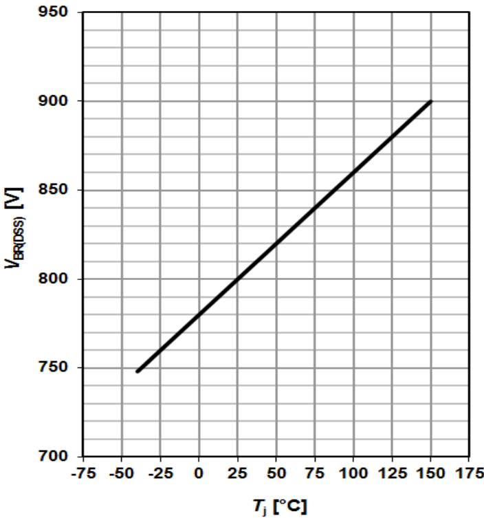
图 24 ICE5ARxx80BZS 的漏源击穿电压； V_{BR(DSS)}=f(T_J) ， I_D=1\text{ mA}
