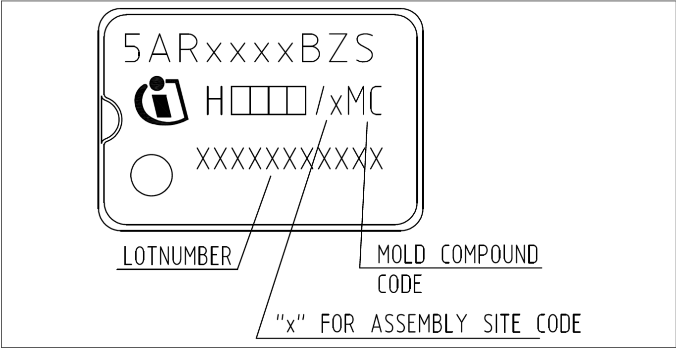
图 32 PG-DIP-7 标记
