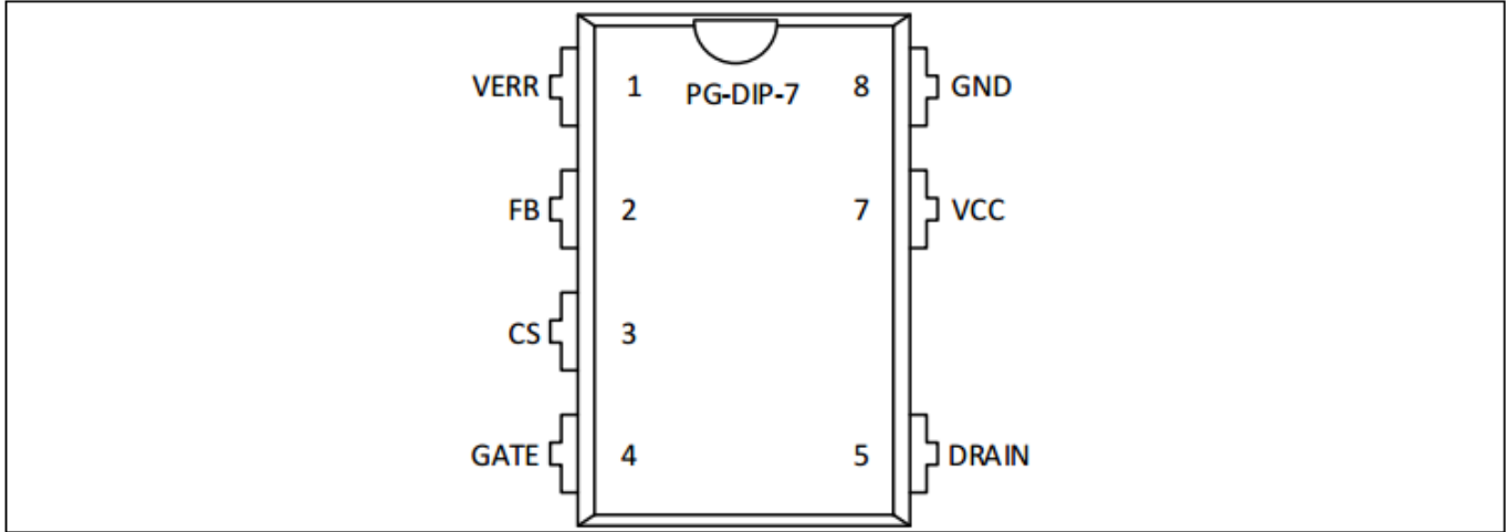
图 3 引脚配置
