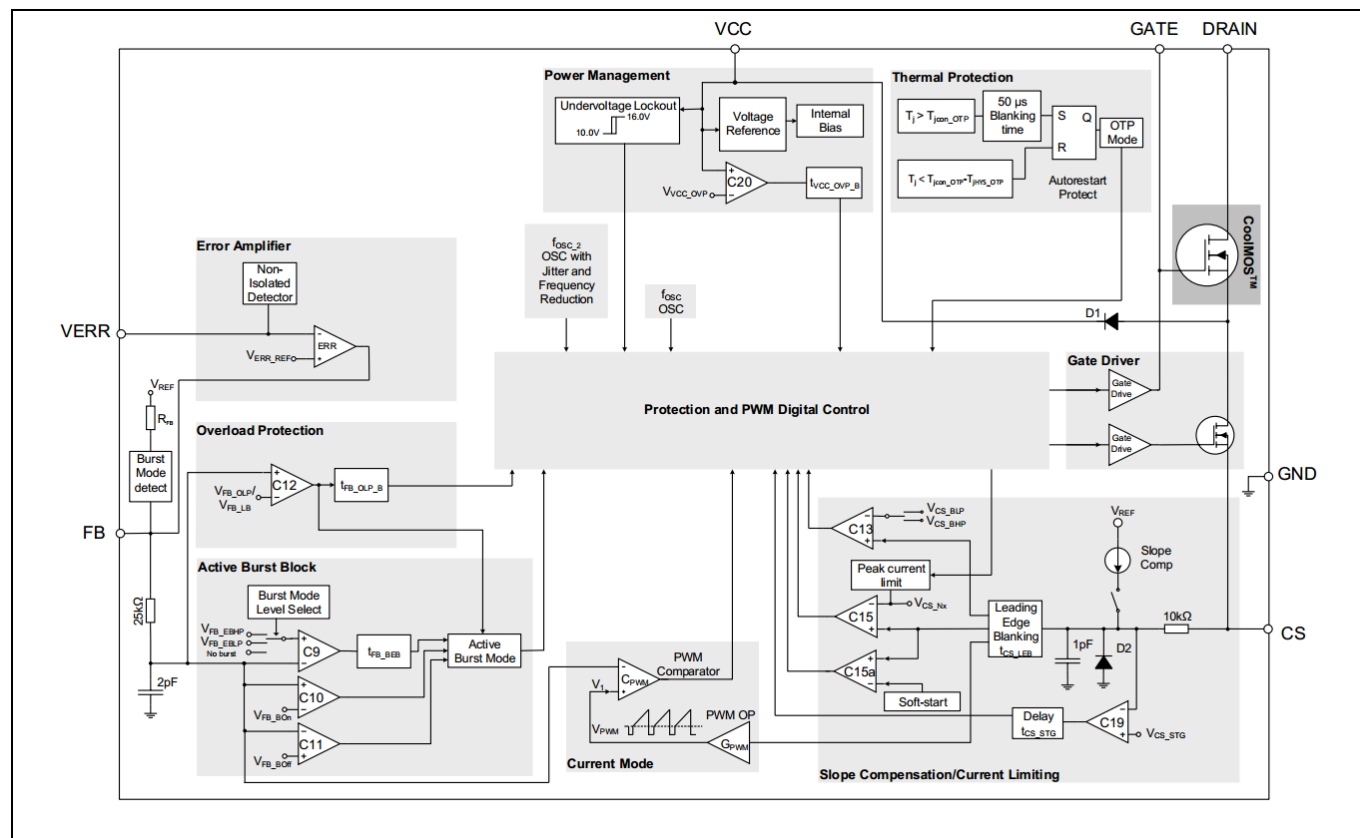
图 4 示例框图
