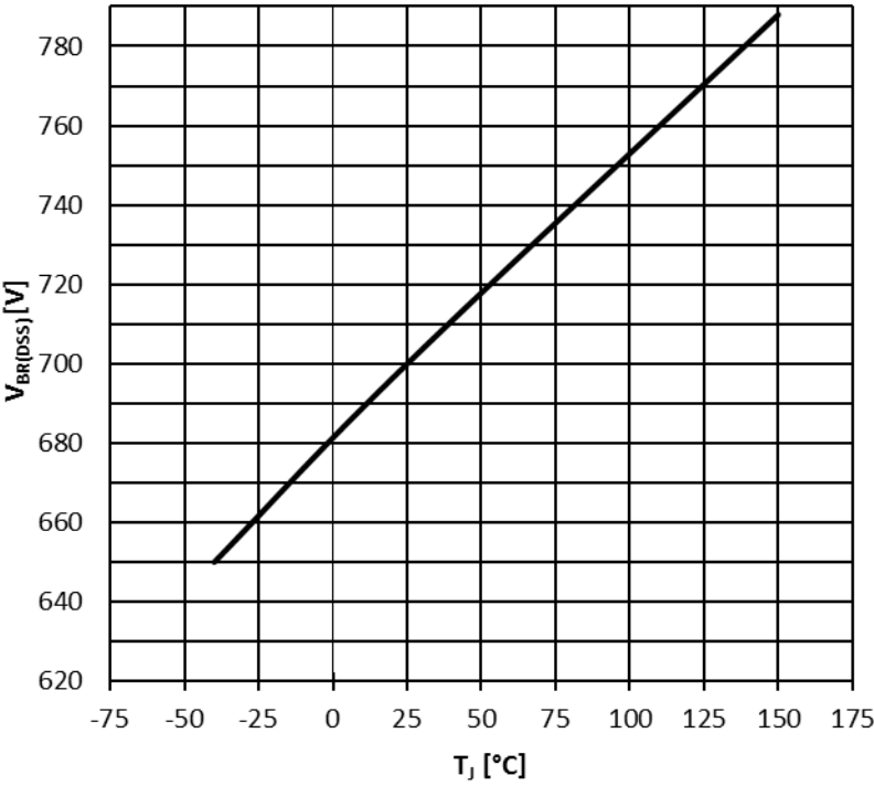
图 23 ICE5ARxx70BZS 的漏源击穿电压； V_{BR(DSS)}=f(T_J) ， I_D=1\text{ mA}
