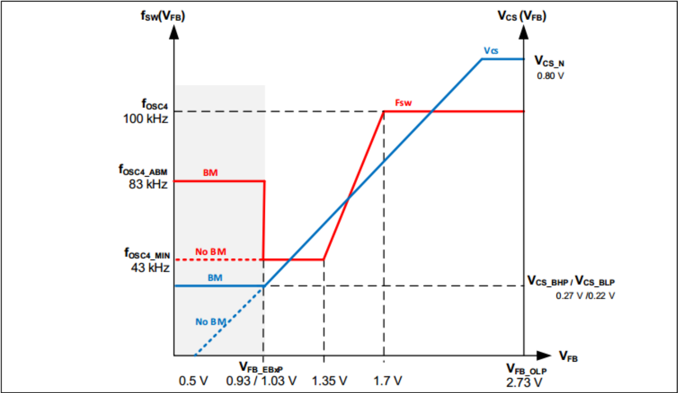
图 8 降频曲线
