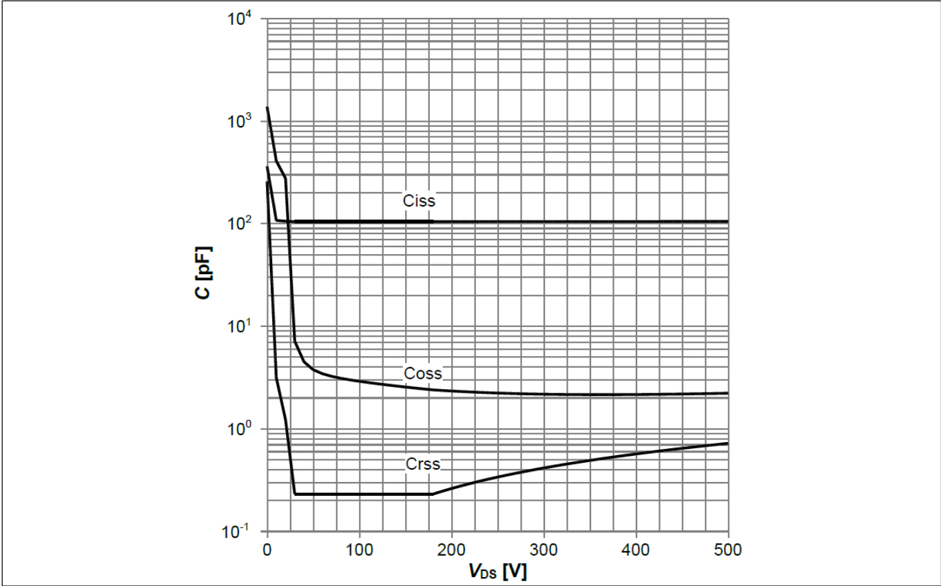
图 26 ICE5AR4780BZS 的典型 CoolMOS™ 电容 ( C=f(V_{DS}) ; V_{GS}=0 V; f=250 kHz)
