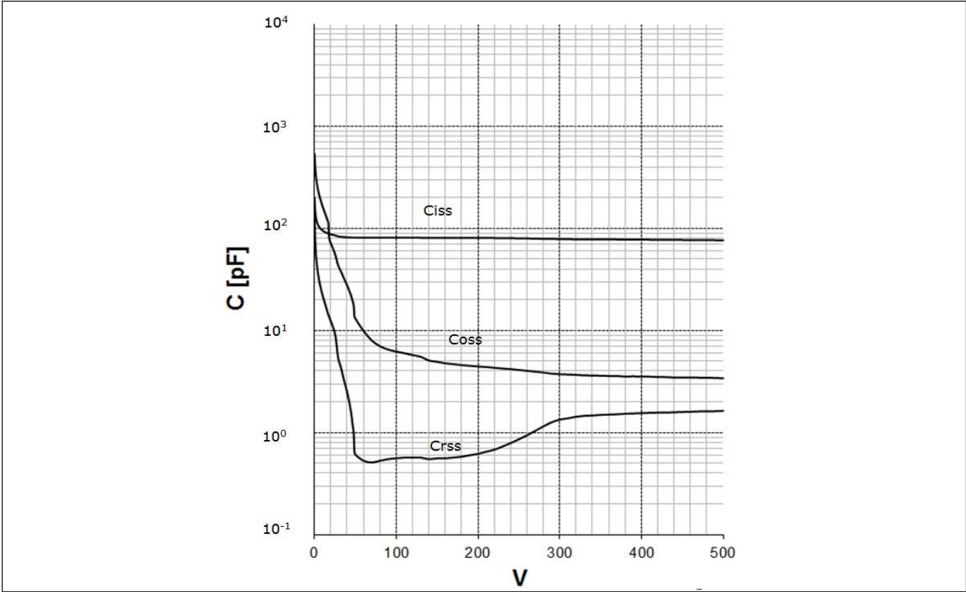
图 25 ICE5AR4770BZS 的典型 CoolMOS™ 电容 ( C=f(V_{DS}) ; V_{GS}=0 V; f=1 MHz)
