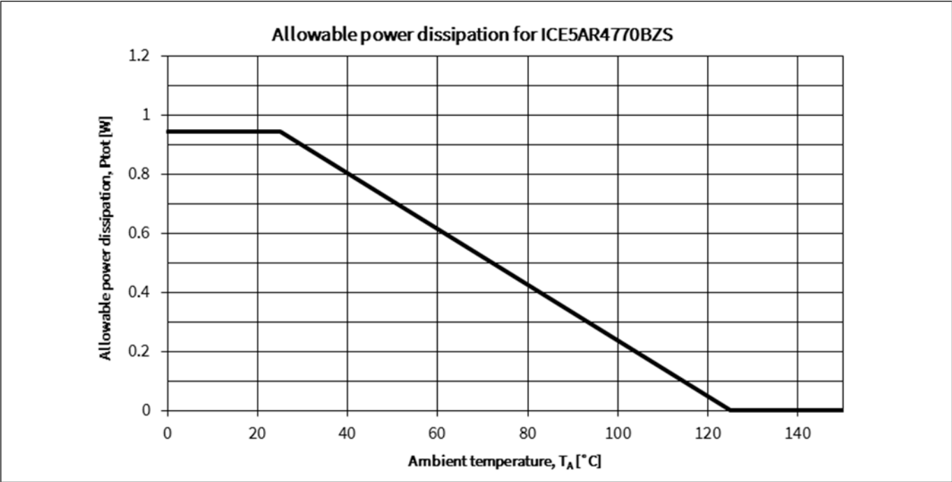
图 20 ICE5AR4770BZS 的功率耗散； P_{\text{tot}}=f(T_a) ，（不得超出第 4.1 节中给出的最大额定值）
