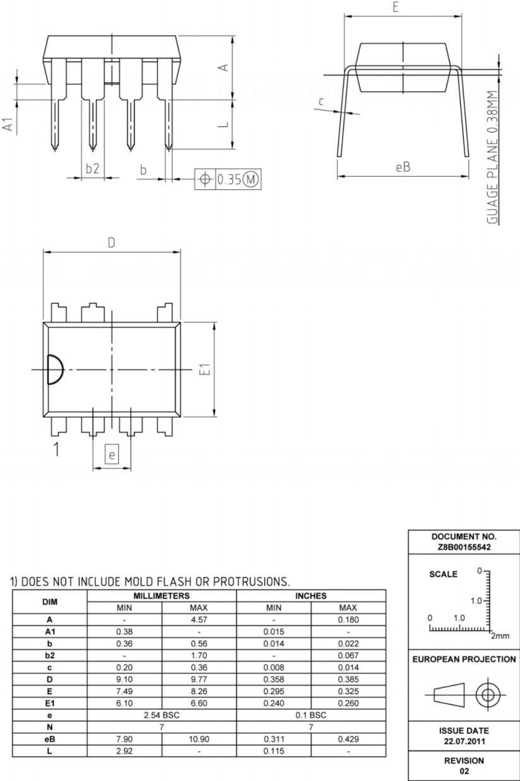
图 31 PG-DIP-7
