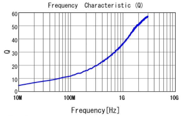
■ LQG15HS1N5B02 Q
