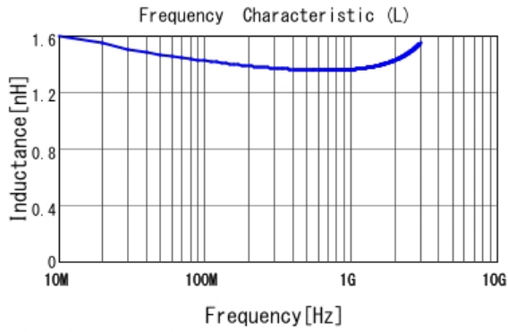
■ LQG15HS1N5B02 L
