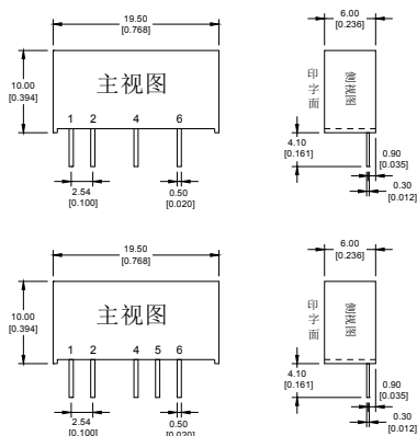
封装尺寸图
