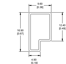
注: 单位 (Unit) : mm[inch] 未注明公差: x.x±0.5mm[x.x±0.020inch] 0.x±0.2mm[x.x±0.008inch] 管长: 220mm[8.66inch] 包装数量: 10pcs 内盒: 235*160*82mm 包装: 9管*5层 外箱: 335*225*280mm 包装: 6盒*1箱
