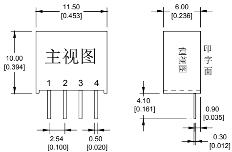
封装尺寸图
