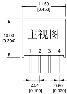
封装尺寸图
