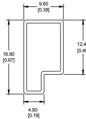
注： 单位 (Unit) : mm[inch] 未注明公差: x.x±0.5mm[x.x±0.020inch] 0.x±0.2mm[x.x±0.008inch] 管长: 220mm[8.66inch] 包装数量: 17pcs 内盒: 235*160*82mm 包装: 9管*6层 外箱: 335*225*280mm 包装: 6盒*1箱
