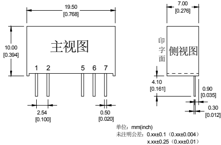
封装尺寸图
