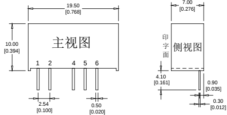
封装尺寸图
