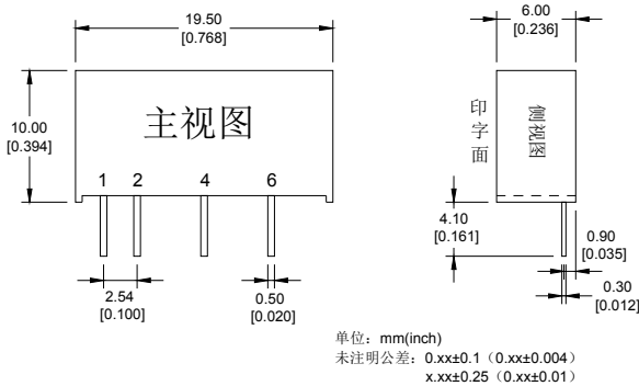
封装尺寸图
