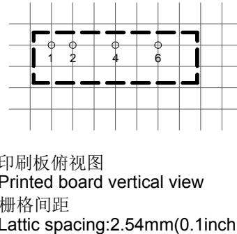
建议印刷板图
