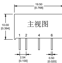
封装尺寸图
