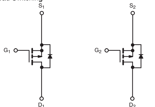
P-Channel MOSFET
