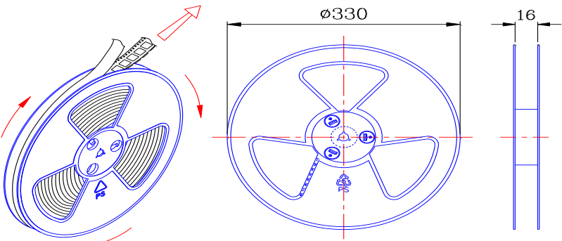
1 Reel : 3000PCS
