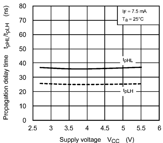
Fig. 12.2.17 t_{pHL}/t_{pLH} - V_{CC}
