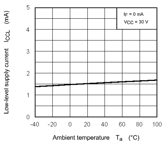
Fig. 12.2.5 I_{CCL} - T_a
