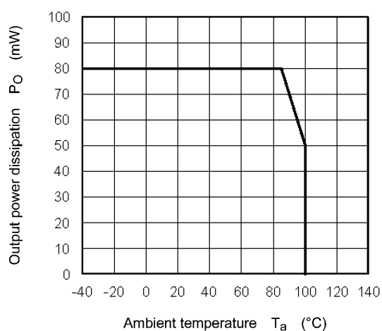
Fig. 12.2.3 P_O - T_a
