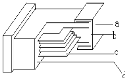
内部结构图:
