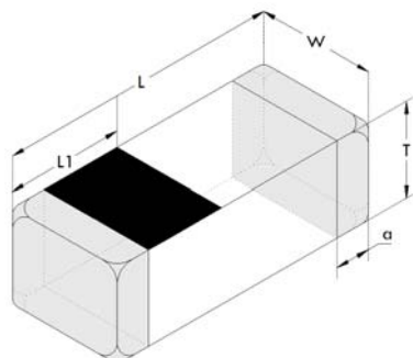
外形尺寸图:
