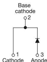
VS-20ETS..
