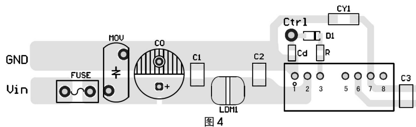
注: 输入输出地之间(CY)焊盘最小距离要保证 \geq 2\text{mm} 。
