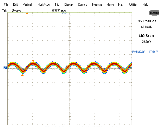
Fig. 20. Output Voltage Ripple, 2A load Ch 2 : V_o
