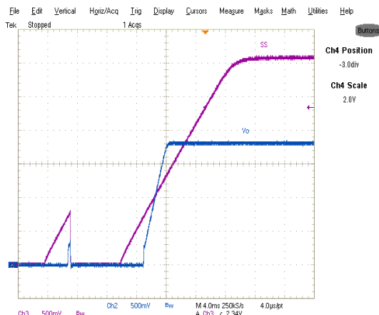
Fig. 22. Short (Hiccup) Recovery Ch 2 : V_o , Ch 3 : V_{ss}
