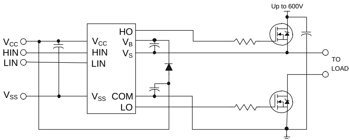
IRS21864(S)
