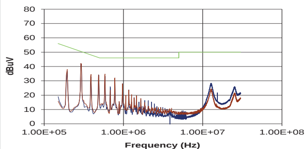
MGJ6D12XXXXWMC (Average)
