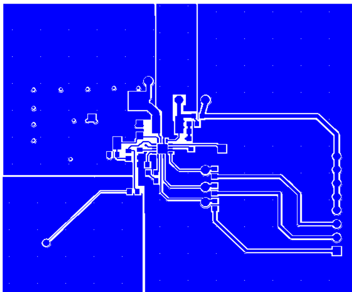
PCB TOP
