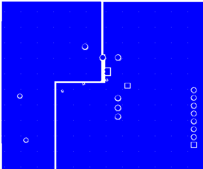
PCB BOTTOM
