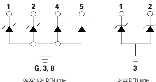
0802/1004 DFN array
