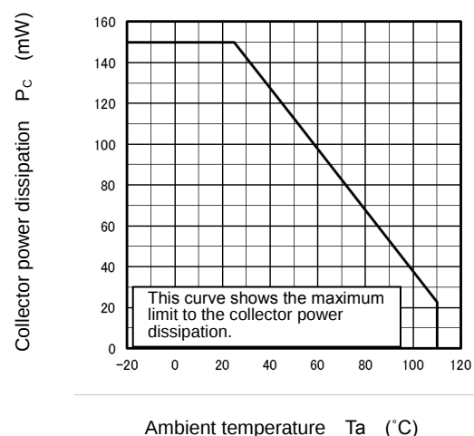
P_C - T_a
