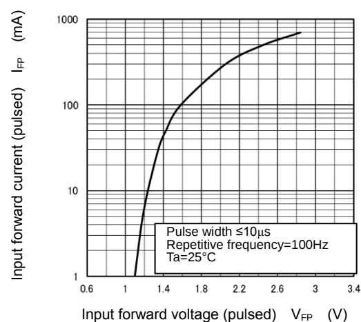
I_{FP} - V_{FP}
