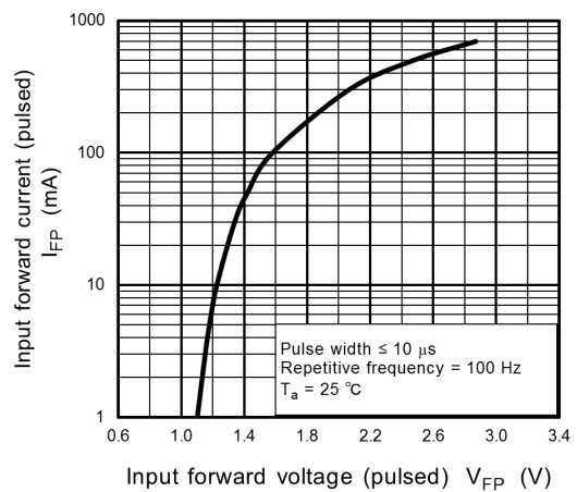
Fig. 11.6 I_{FP} - V_{FP}
