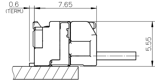
嵌合図
