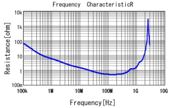
■ DE1E3KX102MB4BN01F R DCOV, 20degC
