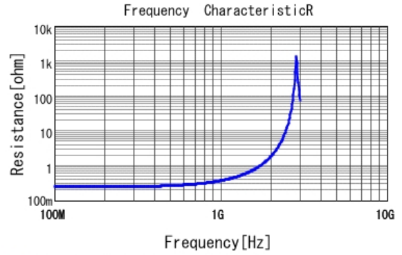
■ DE21XKY470JA2BM01F R DCOV, 20degC
