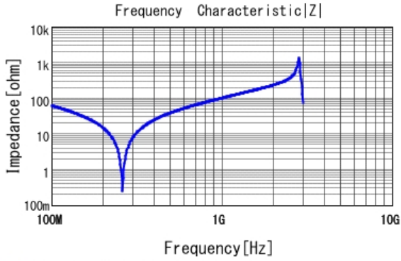
■ DE21XKY470JA2BM01F |Z| DCOV, 20degC
