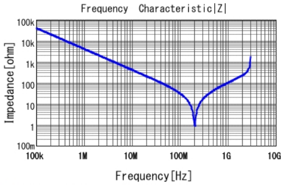
■ DE2B3KY101KA3BU02F |Z| DCOV, 20degC
