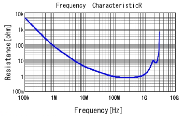
■ DE2B3KY101KA3BU02F R DCOV, 20degC
