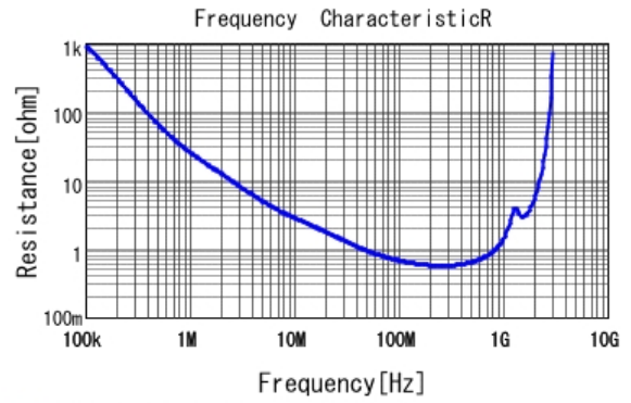
■ DE2B3KY221KA2BM01F R DCOV, 20degC
