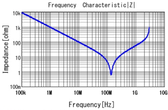
■ DE2B3KY221KA2BM01F |Z| DCOV, 20degC
