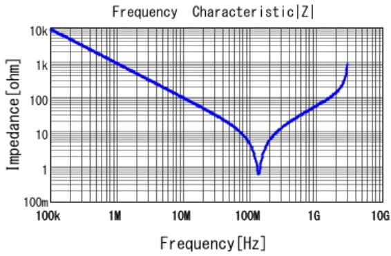
■ DE2B3KY221KA3BM02F |Z| DCOV, 20degC
