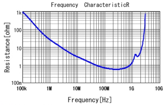
■ DE2B3KY221KA3BM02F R DCOV, 20degC
