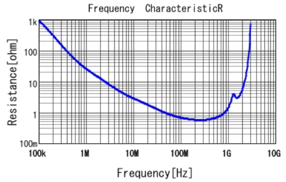
■ DE2B3KY221KB3BU02F R DCOV, 20degC
