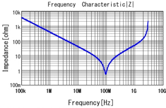
■ DE2B3KY471KA2BM01F |Z| DCOV, 20degC
