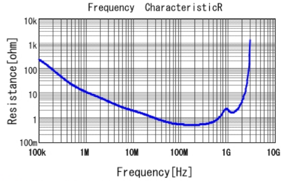
■ DE2B3KY471KA2BM01F R DCOV, 20degC
