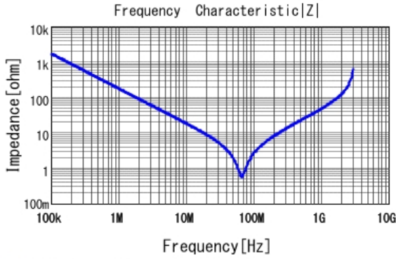
■ DE2E3KY102MA3BU02F |Z| DCOV, 20degC
