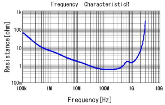
■ DE2E3KY102MA3BU02F R DCOV, 20degC
