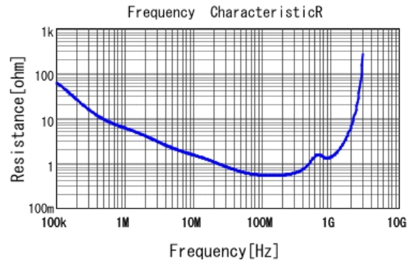
■ DE2E3KY102MN3AM02F R DCOV, 20degC
