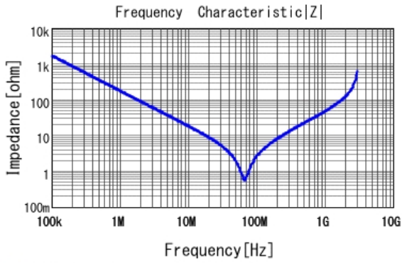
■ DE2E3KY102MN3AM02F |Z| DCOV, 20degC
