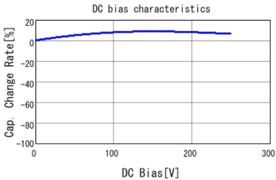
■ DE2E3KY102MN3AM02F C-DC bias capchange, 20.0degC, AC1
