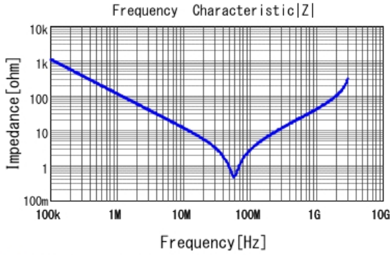
■ DE2E3KY152MA2BM01F |Z| DCOV, 20degC
