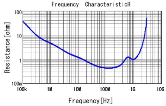
■ DE2E3KY152MA2BM01F R DCOV, 20degC
