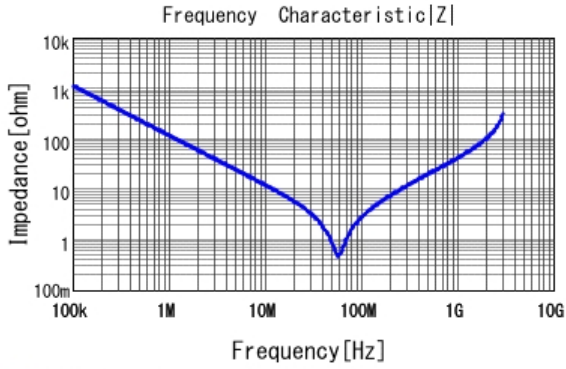
■ DE2E3KY152MN3AM02F |Z| DCOV, 20degC
