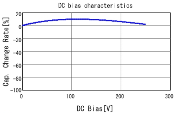
■ DE2E3KY152MN3AM02F C-DC bias capchange, 20.0degC, AC1
