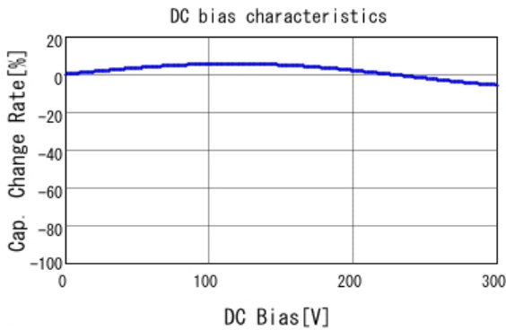
■ DE2E3KY222MN3AU02F C-DC bias capchange, 20.0degC, AC1
