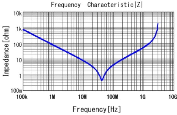
■ DE2E3KY222MN3AU02F |Z| DCOV, 20degC
