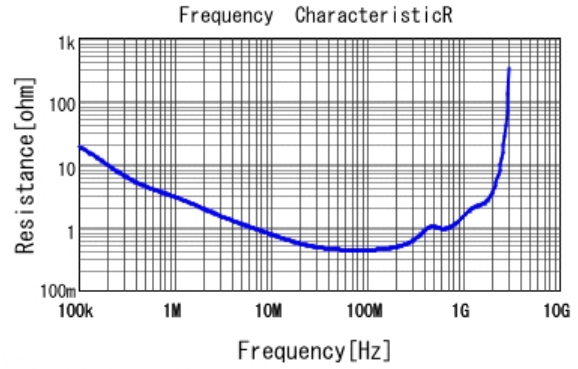
■ DE2E3KY222MN3AU02F R DCOV, 20degC
