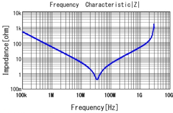
■ DE2E3KY332MA3BM02F |Z| DCOV, 20degC
