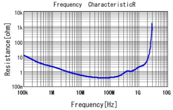
■ DE2E3KY332MA3BM02F R DCOV, 20degC
