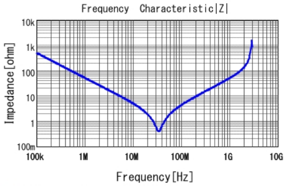
■ DE2E3KY332MA3BU02F |Z| DCOV, 20degC
