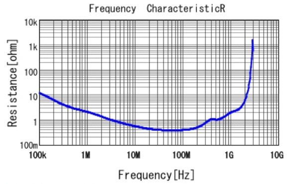
■ DE2E3KY332MA3BU02F R DCOV, 20degC
