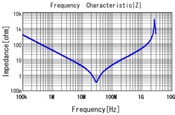
■ DE2E3KY472MA3BU02F |Z| DCOV, 20degC
