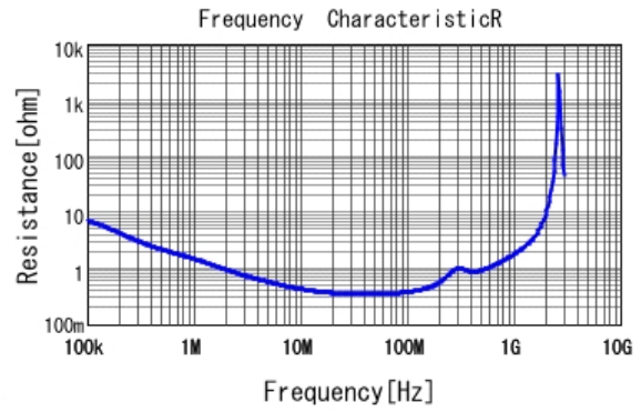
■ DE2E3KY472MA3BU02F R DCOV, 20degC
