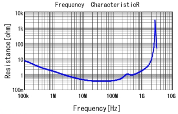
■ DE2E3KY472MB3BU02F R DCOV, 20degC
