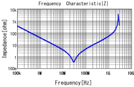
■ DE2E3KY472MN3AU02F |Z| DCOV, 20degC
