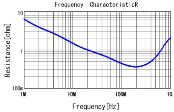
■ DE2E3SA102MA3BX02F R DCOV, 20degC
