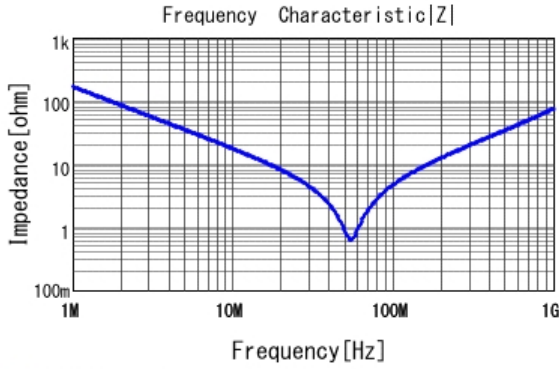
■ DE2E3SA102MA3BX02F |Z| DCOV, 20degC
